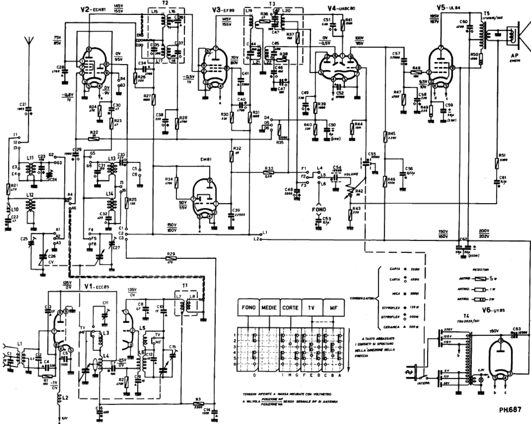
PHONOLA - Mod. 687. Apparecchio per la ricezione delle onde medie e corte a modulazione di ampiezza, e per la ricezione della gamma onde ultracorte sia radio che audio-TV a modulazione di frequenza. Commutazione con tastiera, Occhio magico. Resa d'uscita 4 watt. Consumo 50 watt.
